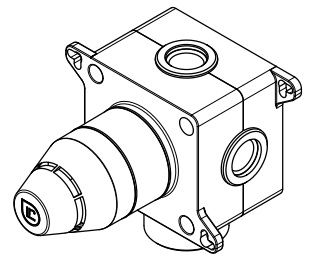
Vista ISO
